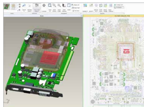
Visuelle Integration von ECAD- und MCAD-Informationen innerhalb einer Benutzerumgebung (erfordert zusätzlich Creo View MCAD).
