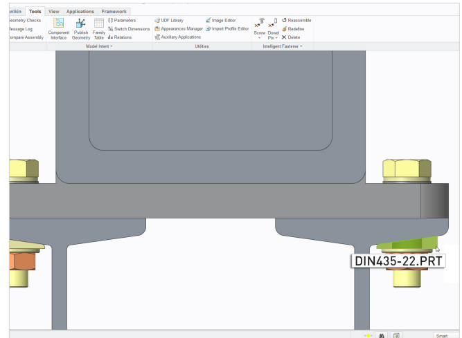
Automatische Ausrichtung von Keilscheiben beim Platzieren
