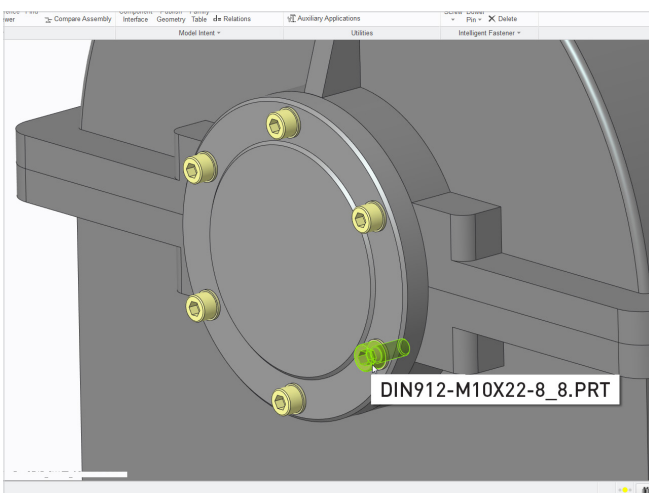
Einbauen von Verbindungselementen auf allen Exemplaren
