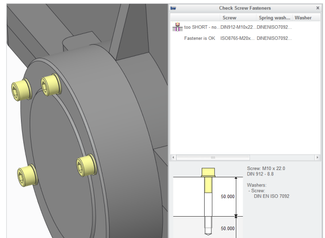
Automatische Validierung
